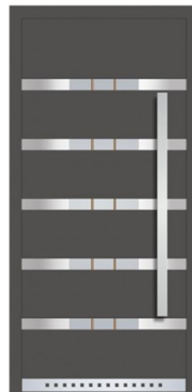
Boja: GRIGIO ANTICO Staklo: TOL Aplikacija: INOX obostrani Rukohvat: DPS 115h Rozeta: RKM 30 Inox zaštita: KZC 100
